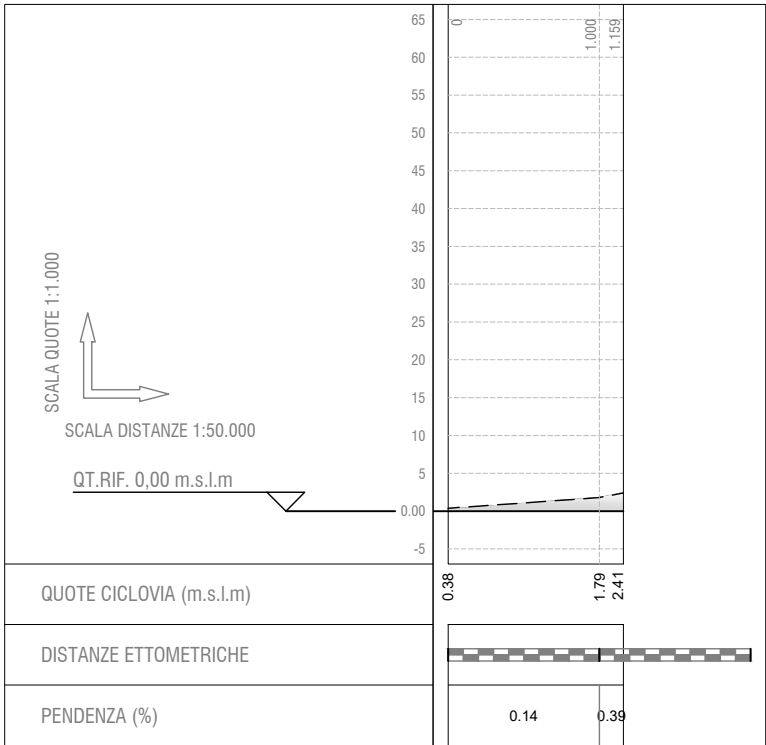
Profilo 6 - Tratto 2.3
