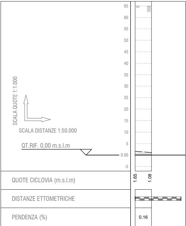
Profilo 5 - Tratto 2.2
